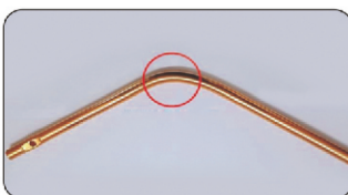
Bend Test Clause 9.7.2 (UL 467)
